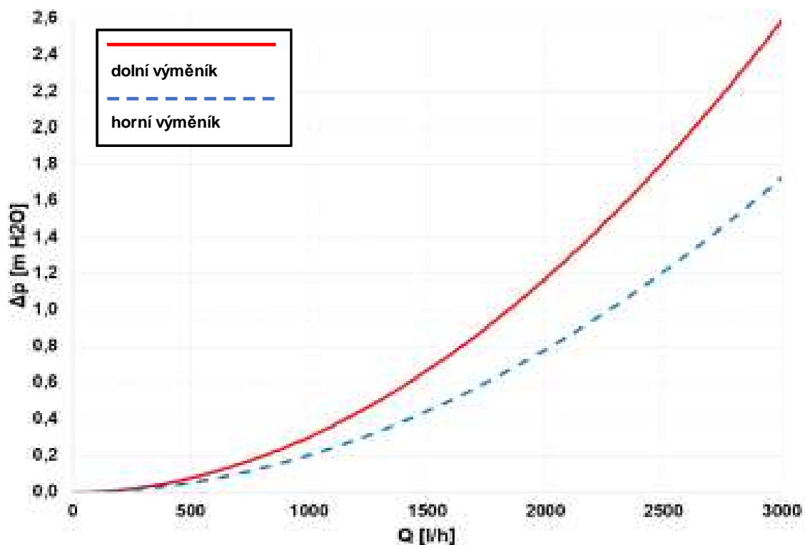
Graf tlakové ztráty výměníku
