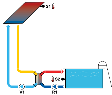
6. Solární systém s výměníkem a bazénem
