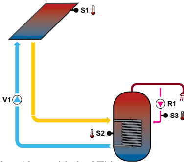
3. Solární systém s cirkulací TV
