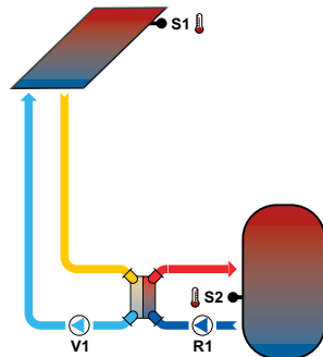
5. Solární systém s výměníkem
